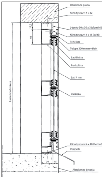
Kiinteän 1-lasisen seinän asennus L-listalla
